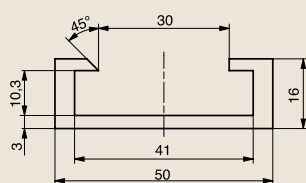
Пластиковый Г-образный профиль для стальной полосы 40 x 8
