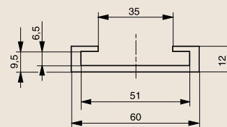
Для стальной полосы 50 x 6 фрезерованный
