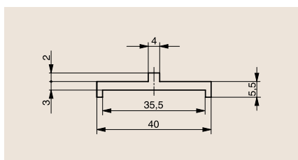
Профиль с утолщением и перемычкой 40 x 7,5
