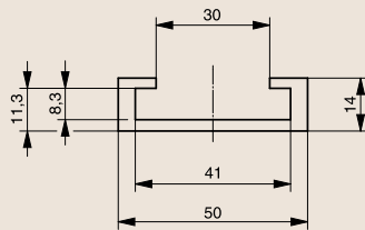
Для стальной полосы 40 x 10 экструдированный
